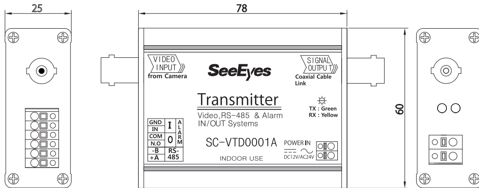
SC-VTD0001A (送信機)
