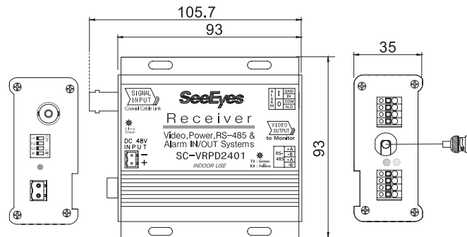
受信機(SC-VRPD2401)
